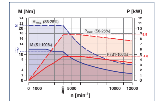
Torretta portautensili BMT45P con motore diretto
