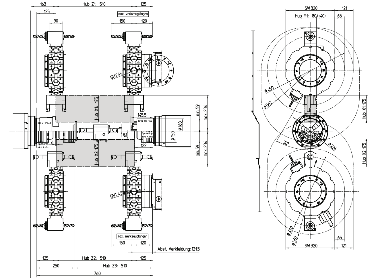
Area di lavoro HT50 con torretta portautensili 12 posizioni BMT45P
