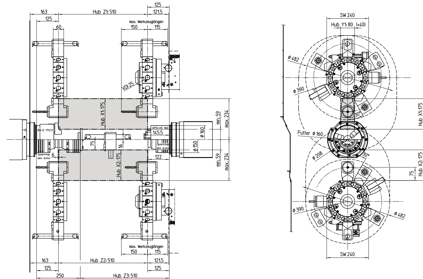
Area di lavoro HT50 con torretta portautensili a 12 posizioni VDI25
