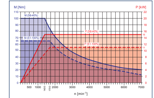
HYPERTURN 50 mandrino principale / contromandrino
