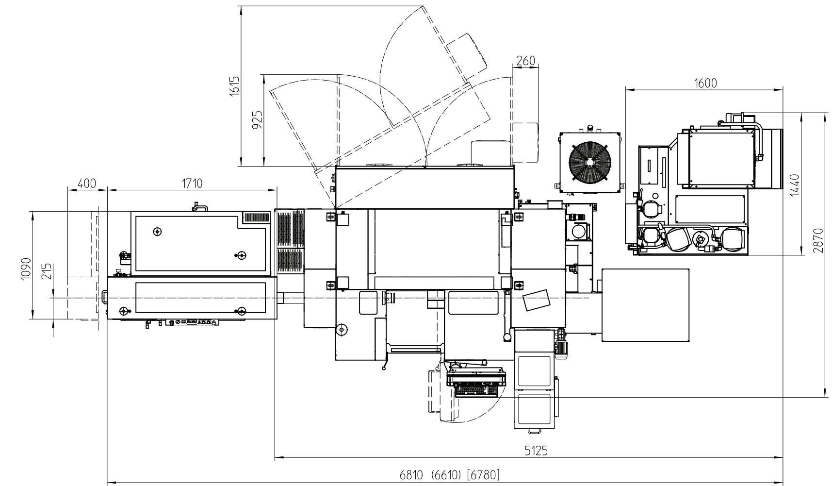
Piano fondazione HT50 con EMCO SL1200 e sistema filtro a carta
