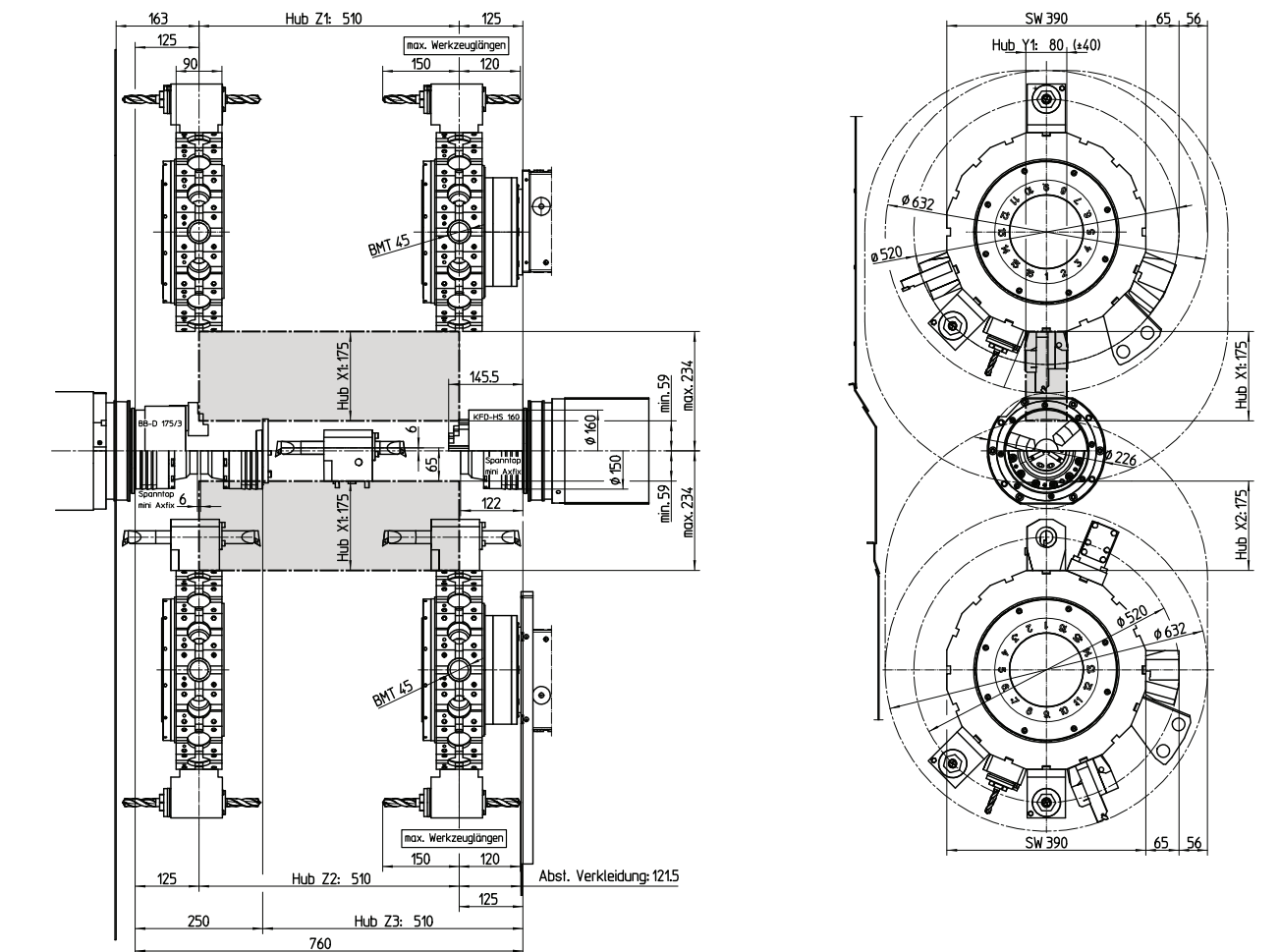
Area di lavoro HT50 con torretta portautensili 16 posizioni BMT45P
